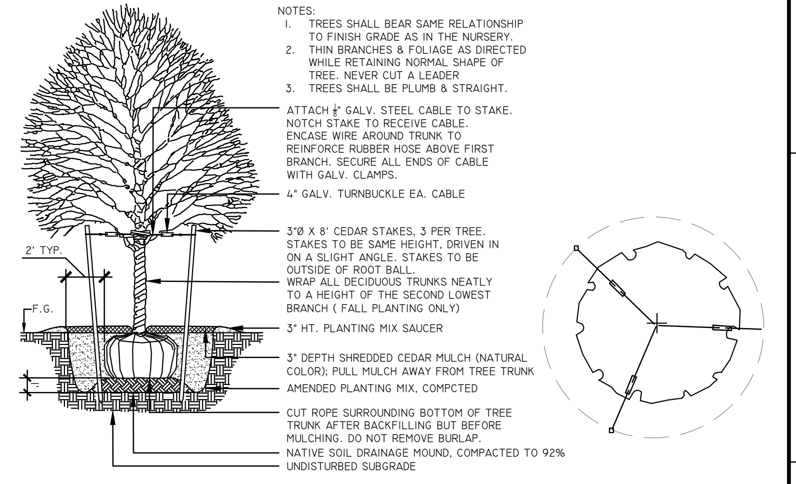
1 DECIDUOUS TREE PLANTING DETAIL SCALE: N.T.S.
