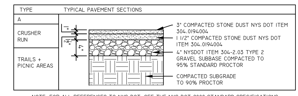
5 ROLLED CRUSHER RUN SCALE: N.T.S.
