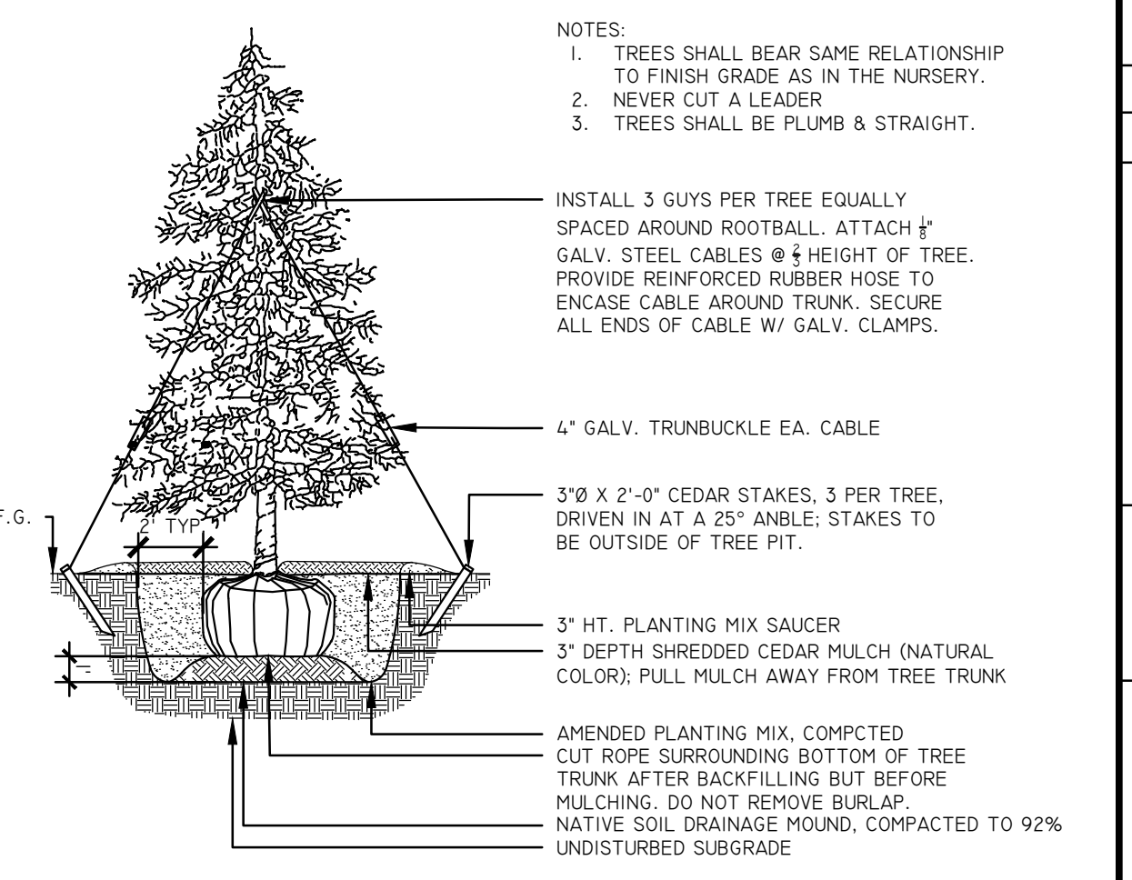
2 EVERGREEN TREE PLANTING DETAIL SCALE: N.T.S.
